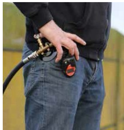
Gasdetektor. Giver alarm ved lys, lyd og vibration når svovlbrintekonzentrationen nærmer sig skadeligt niveau
