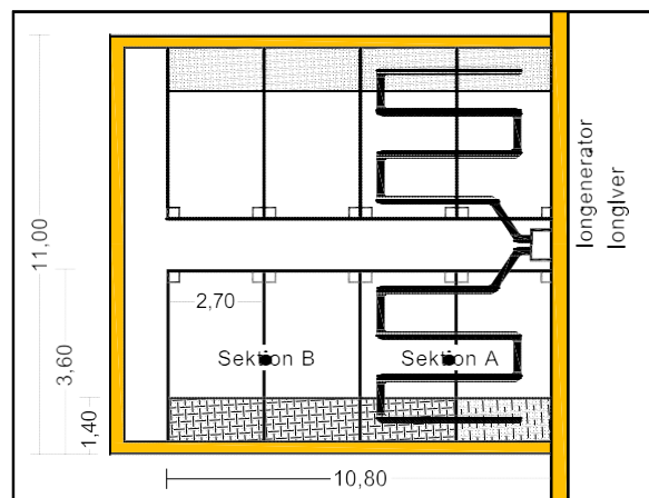
Figur 2. Ioniseringsanlæg
